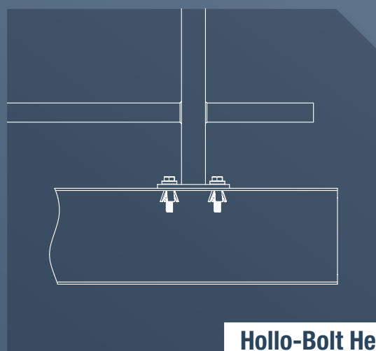
Holo-Bolt HCF
