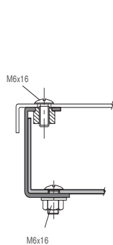
Cable Tray L
